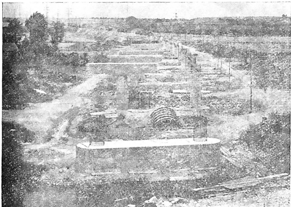
Budování mostních pilířů u Sobětuch
