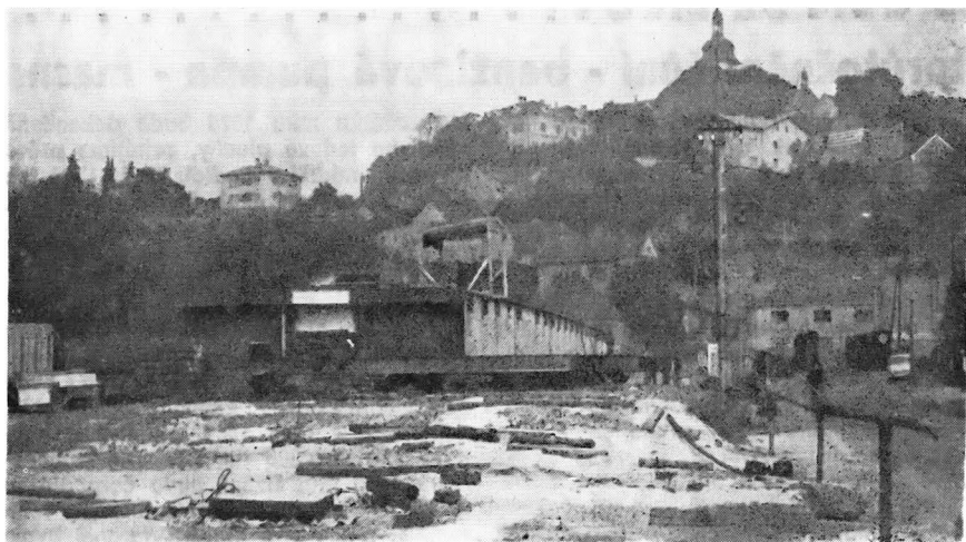
Obsáhlou reportáž z úspěšného usazení mostu ve dnech 9. a 10. října přineseme v listopadovém čísle. Foto J. Antoň, prop. n. p. Karbo
