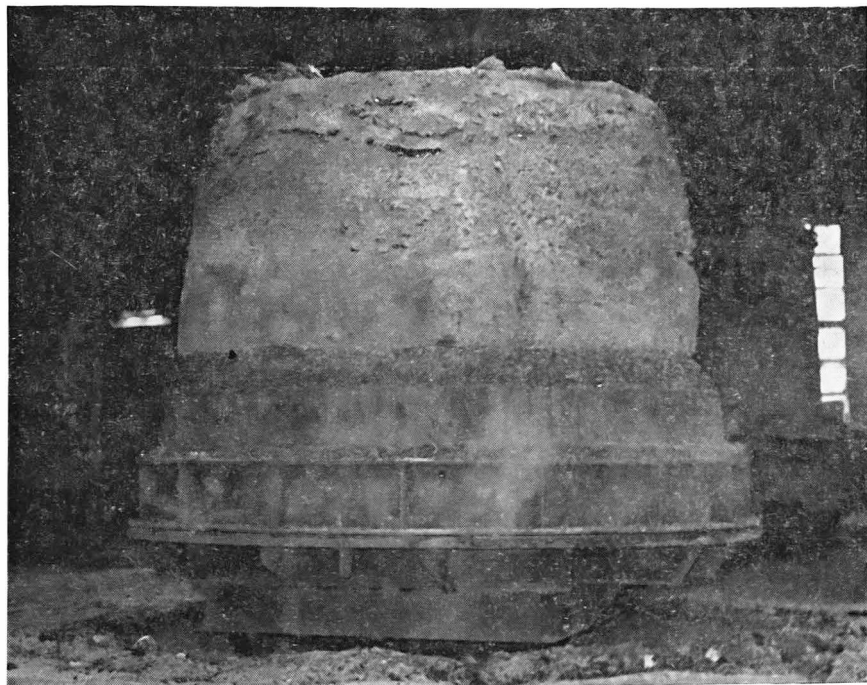
Snímek představuje podvozek pece s vytaveným blokem korundu, v jehož spodní části se feroslitina usazuje.
